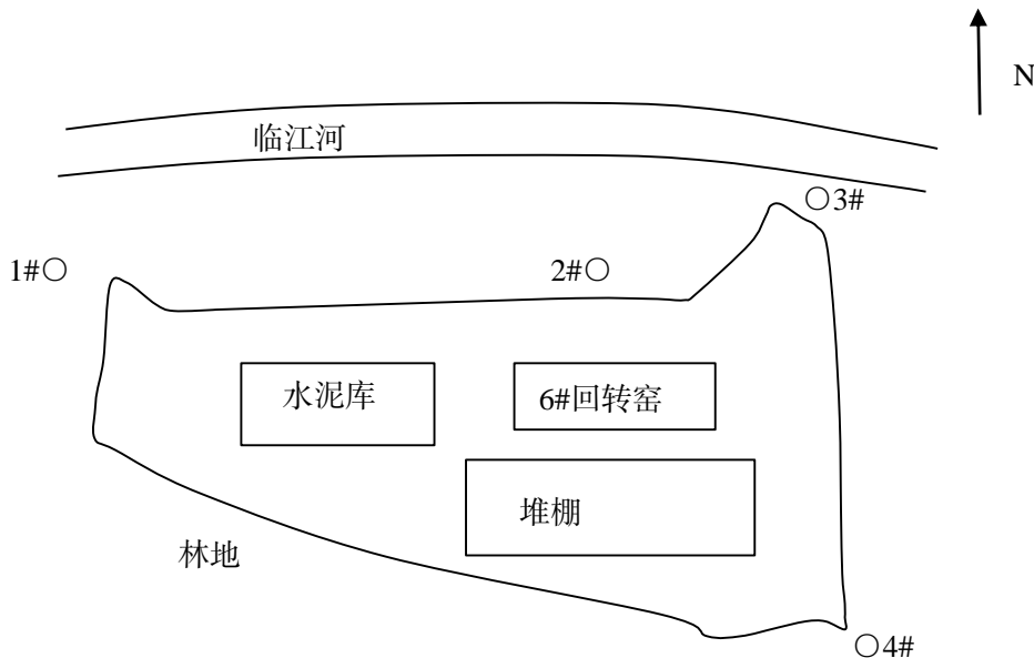
附 1: 六期废气 (无组织) 测点示意图
